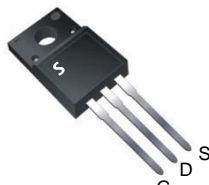
HFS730F TO-220F
